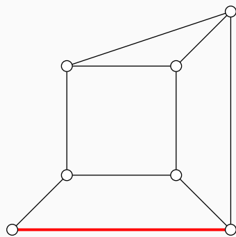
3 контракция на ребро
