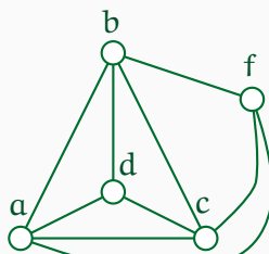
Фигура 2.79 : Алгоритъм, строящ триангулации.
