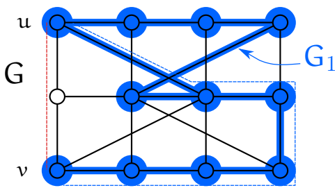
Фигура 2.24: Най-късият път между u и v в G е очертан с червена прекъснатата линия . Най-късият път между u и v в G_1 е очертан със синя прекъснатата линия .
