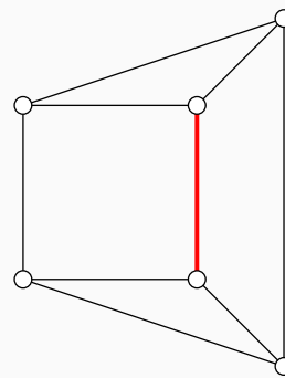
4 контракция на ребро
