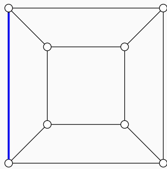
1 изтриване на ребро
