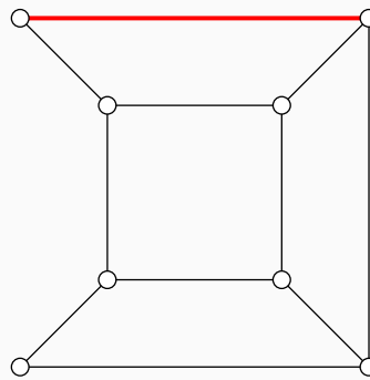
2 контракция на ребро
