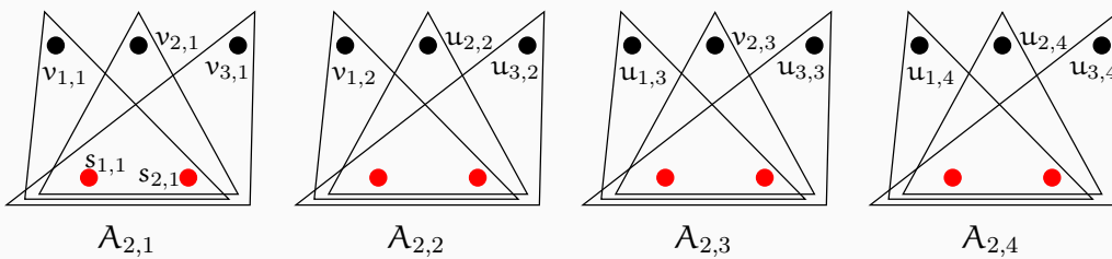
Фигура 16.23 : 3SAT \leq_p 3DM върху екземпляра от (16.10): короните.
