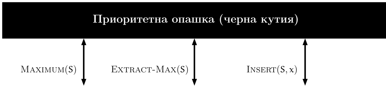
Фигура 5.19: АДТ приоритетна опашка като черна кутия. Конкретната имплементация е скрита. Отвън се “виждат” само трите функции на интерфейса.
