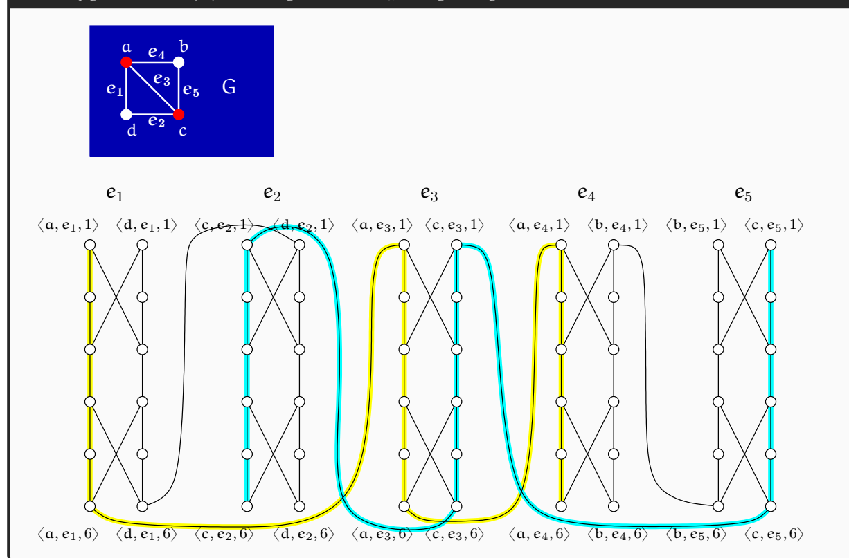
Фигура 16.39 : Двете вериги от P_U в примера.
