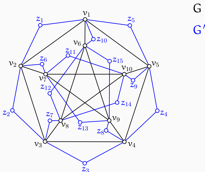
Фигура 16.9 : G и G' от \text{VERTEX COVER} \leq_p \text{DOMINATING SET} .
