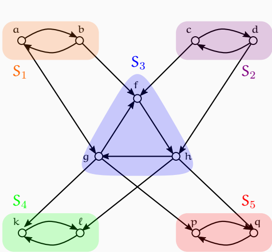
Фигура 9.4 : Различни наредби на V индуцират различни наредби на \text{SCC}(G) .
