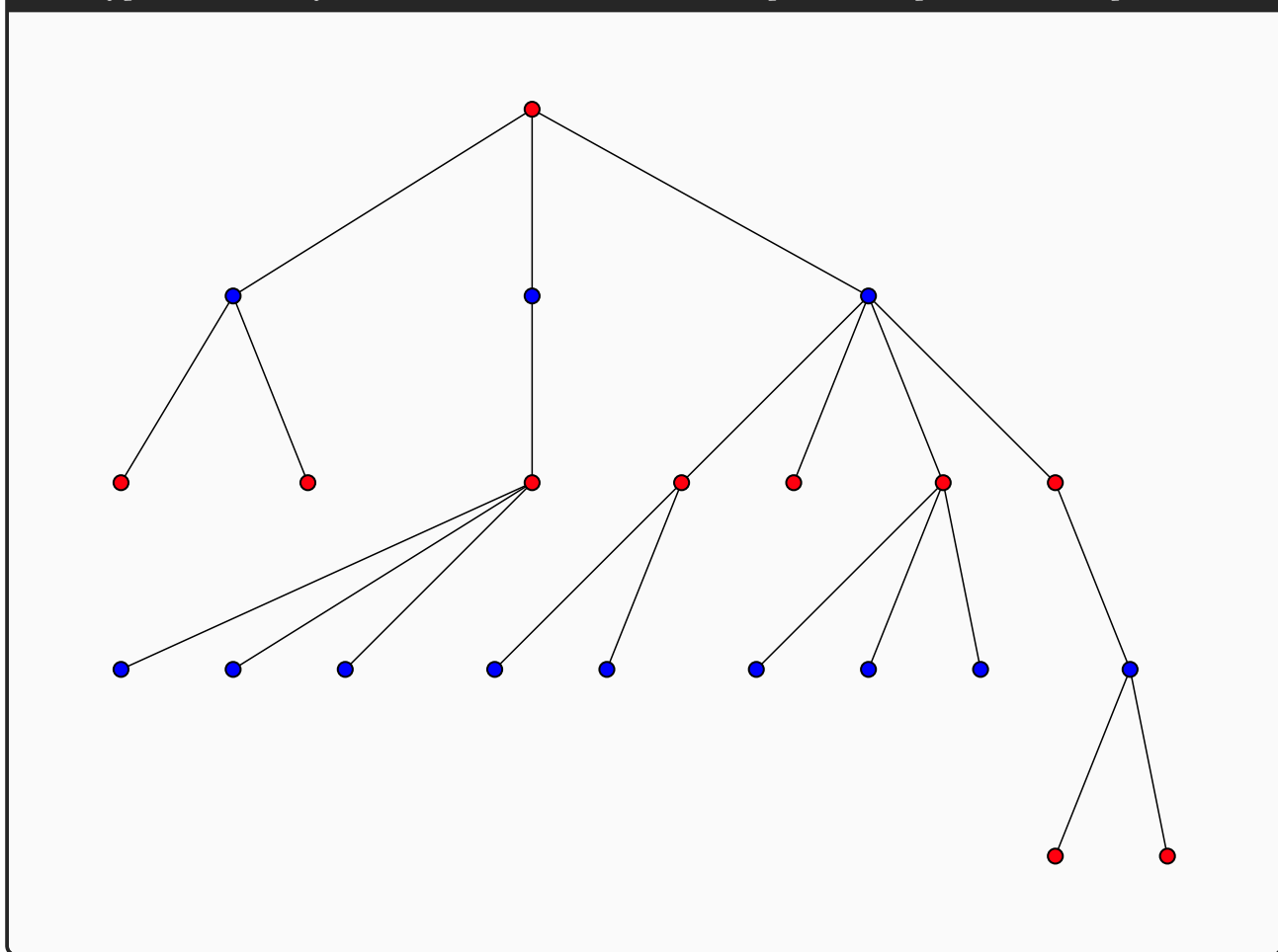
Фигура 12.3 : Редуване на нива не дава мин. върхово покриване на дърво.
