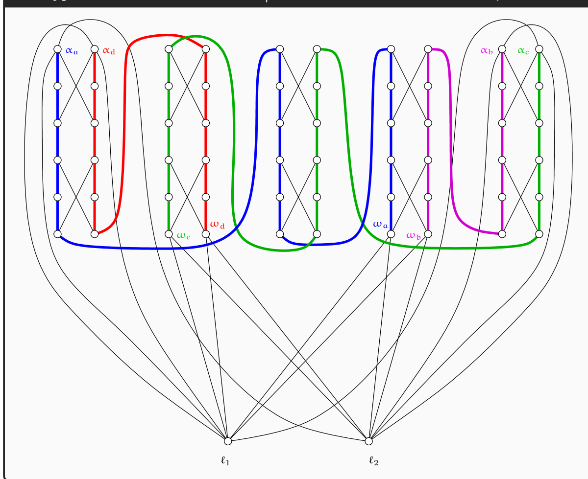
Фигура 16.37 : VERTEX COVER \leq_p HAM. CYCLE: окончателният J.
