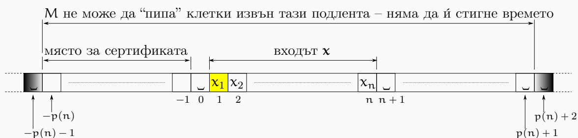
Фигура 15.3 : Началното съдържание на лентата на M(x) в Теорема 135.
