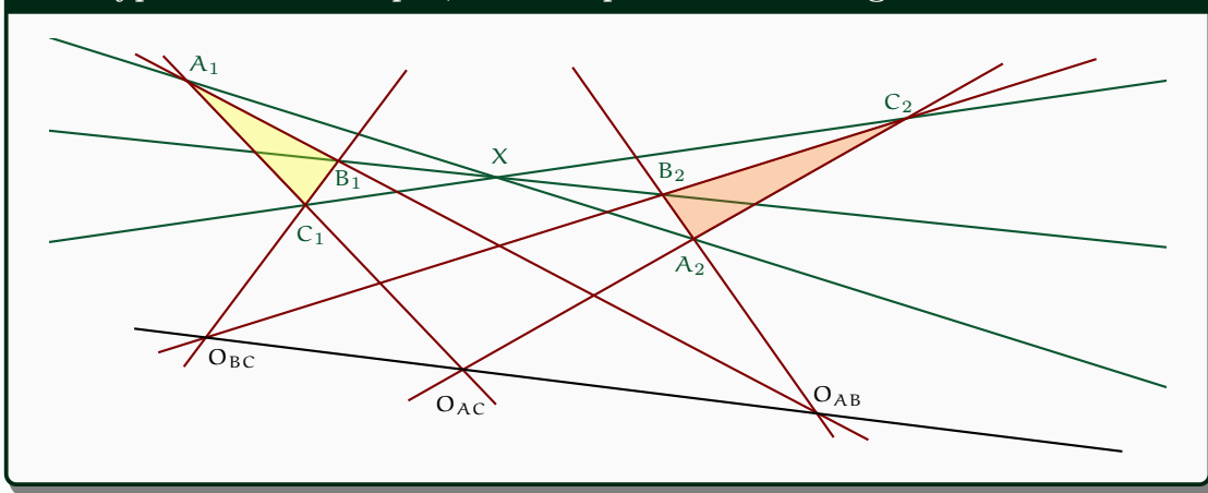
Фигура 2.33 : Илюстрация на теоремата на Desargues.
