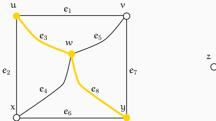
Фигура 2.12 : Графът G_1 от Фигура 2.1 и неговият подграф, индуциран от \{u, w, y\} , оцветен в оранжево.
