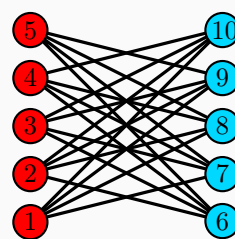
Фигура 2.46(в): 2-оцветяване.
