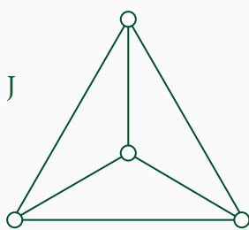
Фигура 2.71 : Ойл. и Хам. цикли в графи и линейните им графи.
