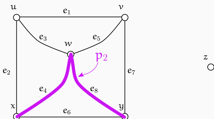
Фигура 2.21 : Прост път p_2 в графа G_1 от Фигура 2.1.
