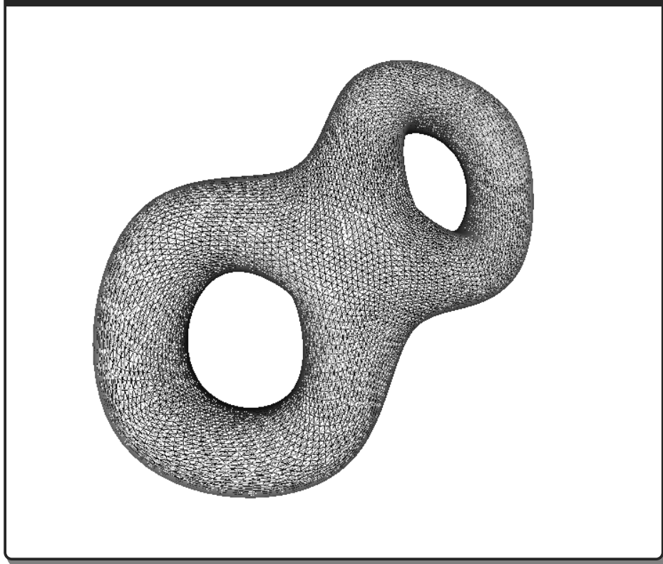
Фигура 2.98 : Wireframe на двоен тороид.
