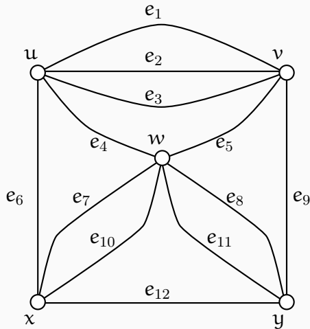
Фигура 2.15 : Пример за неориентиран мултиграф G .
