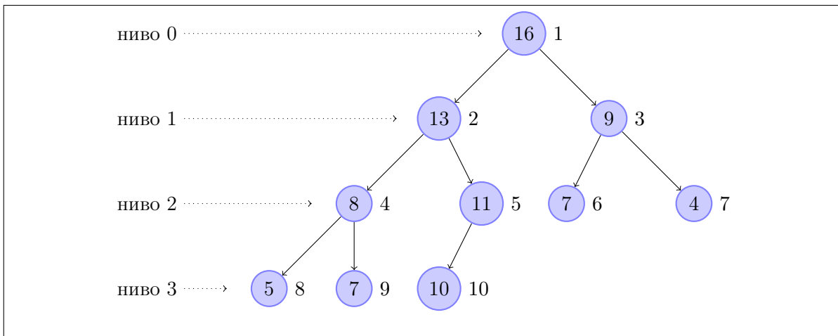
Фигура 2: Пирамида. Във всеки връх е изписана стойността на ключа, а встрани е изписана позицията на върха в масива A .
