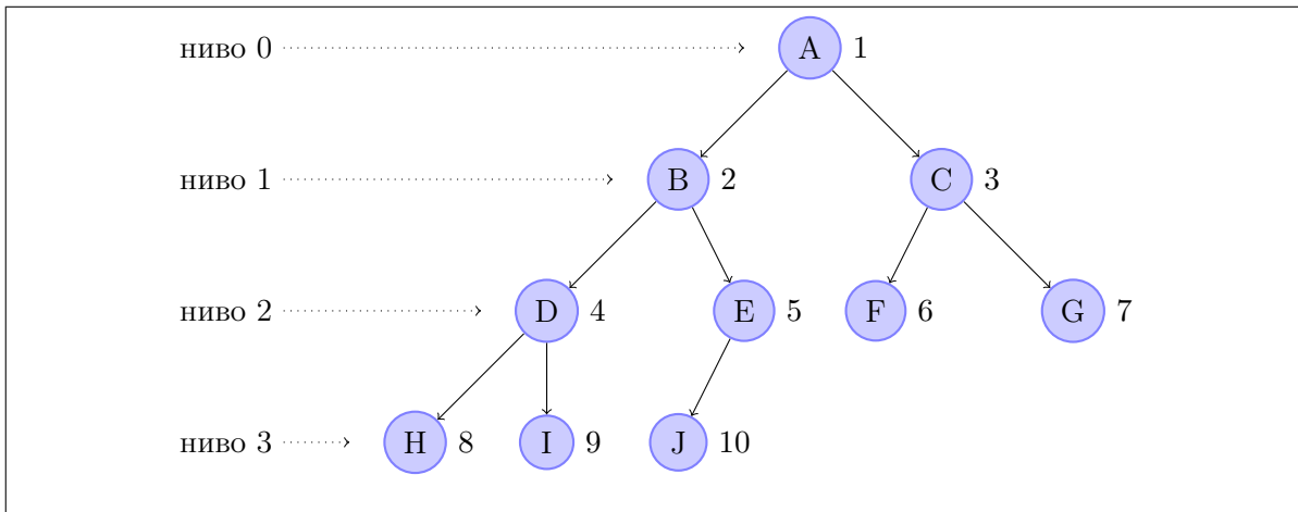
Фигура 1: Попълнено двоично дърво: всички нива са запълнени с изключение на последното, където са запълнени няколко върха плътно в лявата част на нивото.
