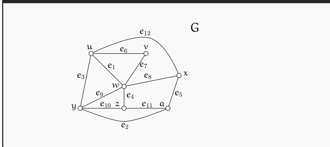
Фигура 16.19 : Граф G .
