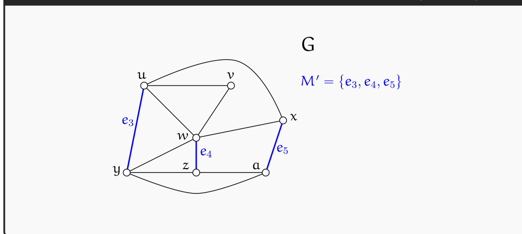
Фигура 16.20 : Максимално по мощност съчетание M' = \{e_3, e_4, e_5\} .
