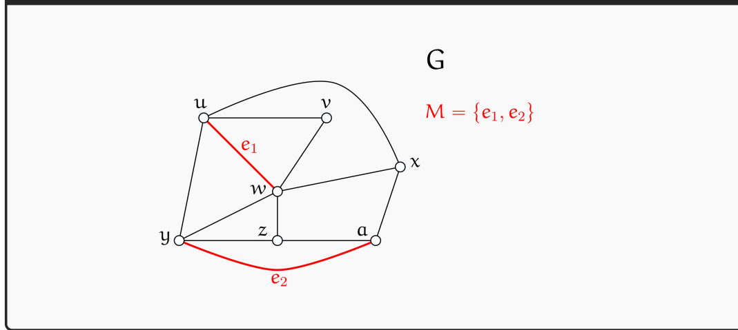
Фигура 16.19 : Максимално по включване съчетание M = \{e_1, e_2\} .
